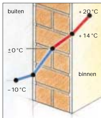
Buitenwand niet geïsoleerd
